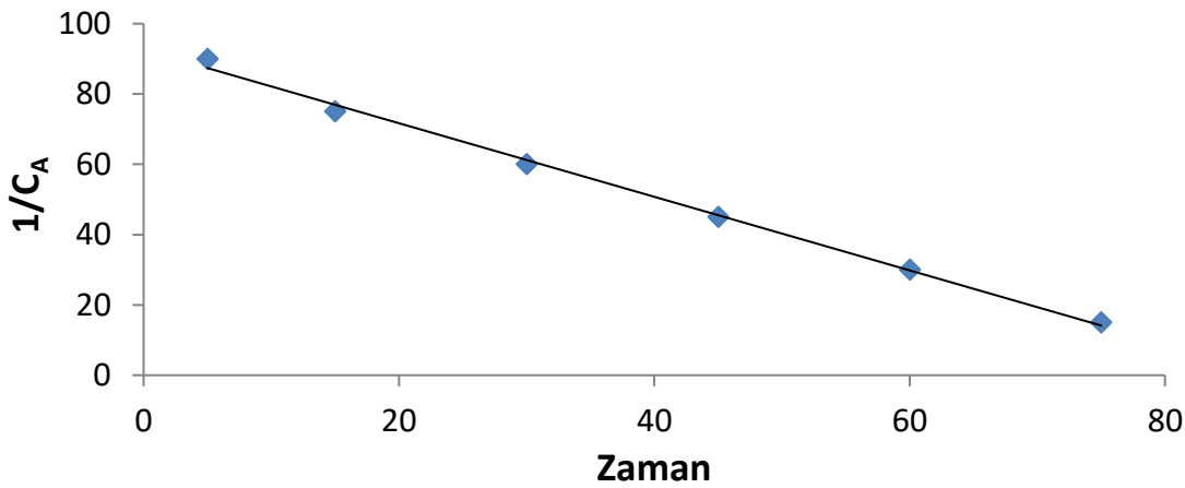
Şekil 4.8.3 İkinci mertebe için 1/C - \text{zaman} grafiği
