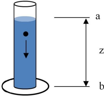
Şekil 4.1.2 Stokes yasaı uyarınca viskozluk tayini [2].
