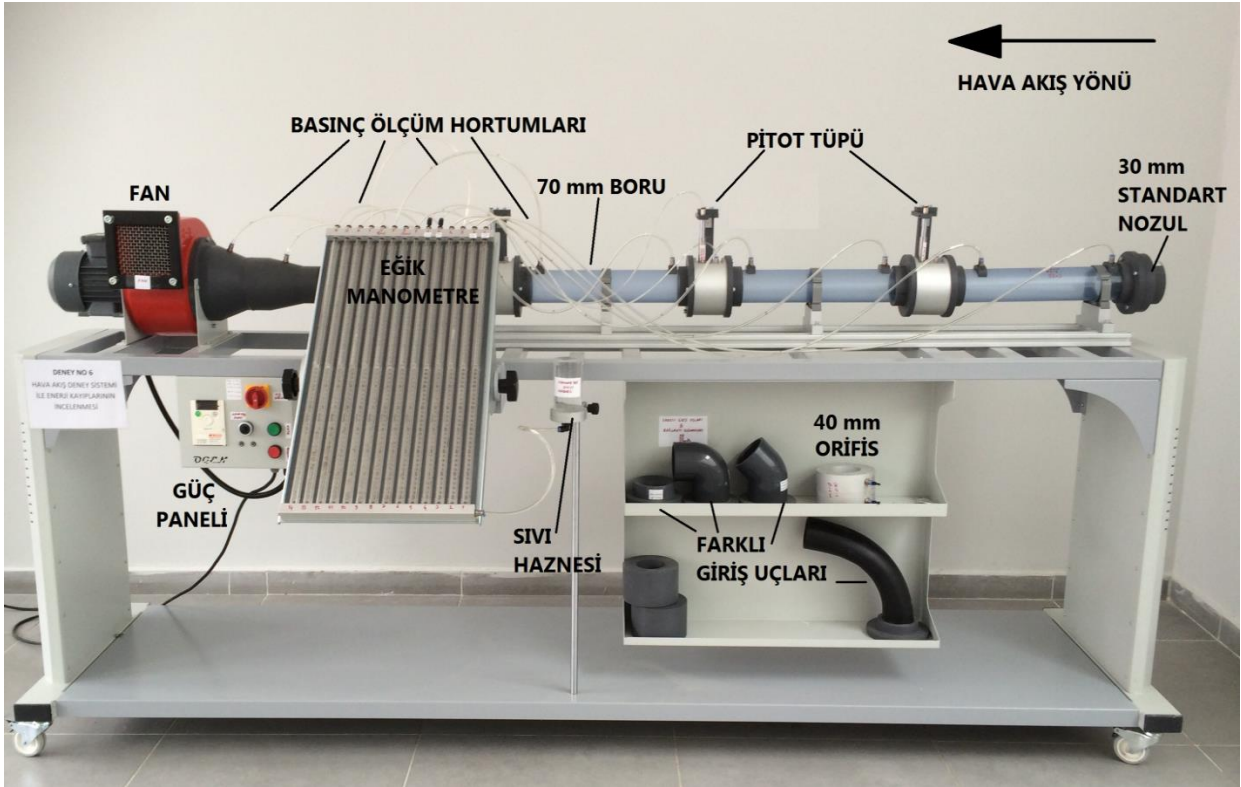
Şekil 11. Hava Akış Deney Düzenneđi
